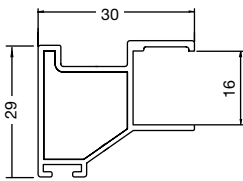
Perfil "U" Aluminio
