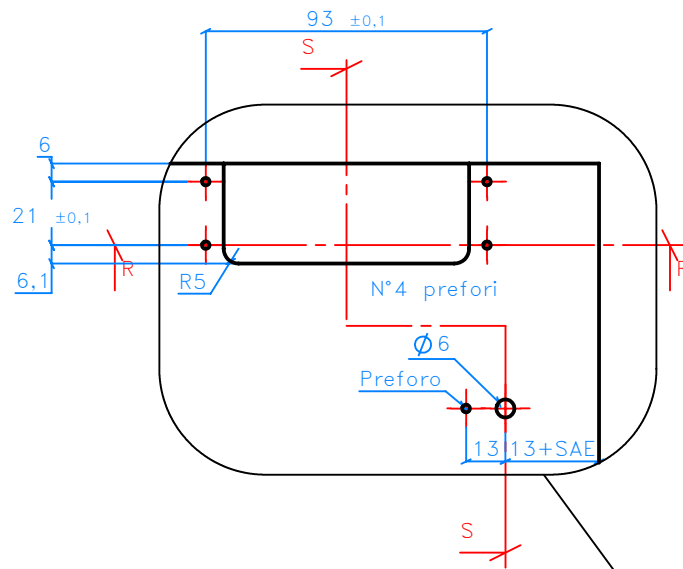
Sez. R-R
