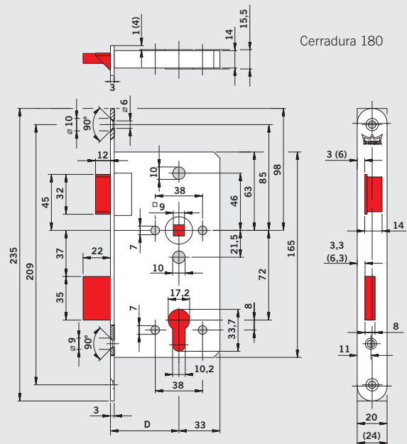
Dibujo DIN-Izquierda (Imagen simétrica DIN-Derecha)
