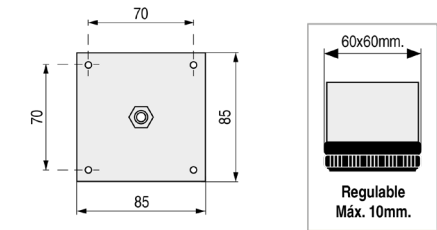
Soporte en hierro acabado zincado
