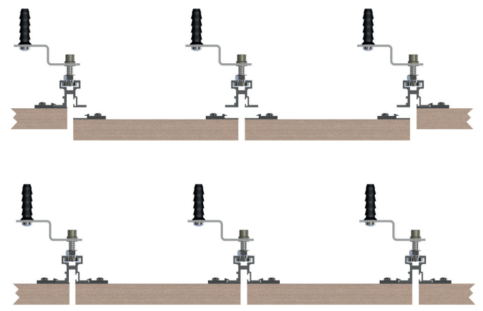
MONTAJE CLIP PANELADO
