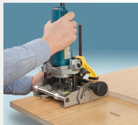
Fresado a 0°
