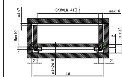
LW 柜体净宽 SKW 抽屉净宽
