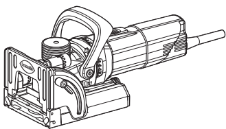
Zeta P2 – Fresadora de ranuras
