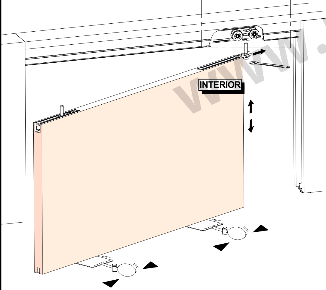
19 MONTAJE PUERTA LADO INTERIOR / Interior side door assembly
