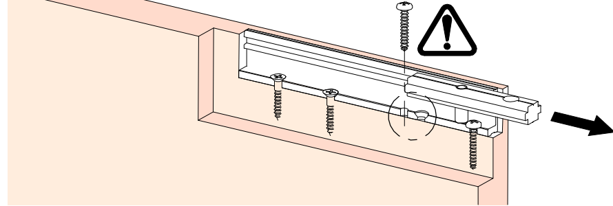
19 MONTAJE PUERTA LADO INTERIOR / Interior side door assembly
