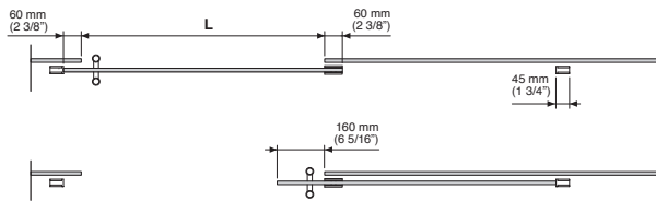
VIDRIO FIJO 10 mm / FIXED GLASS 3/8"
