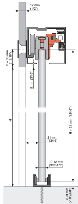
VIDRIO FIJO 12 mm / FIXED GLASS 1/2"
