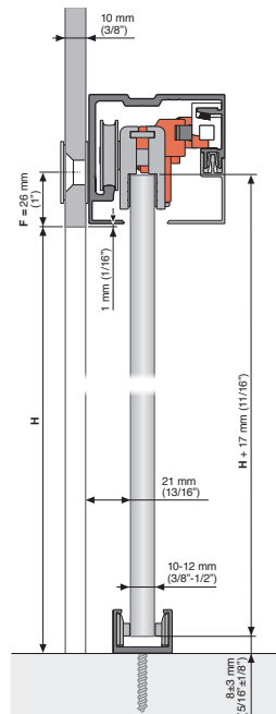
VIDRIO FIJO 10 mm / FIXED GLASS 3/8"
